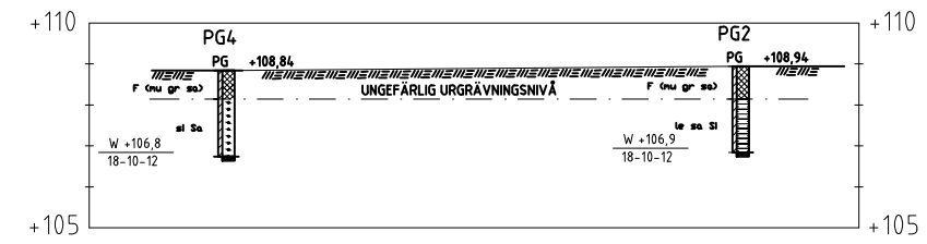
SEKTION A-A, PROVGROP 2, 4
